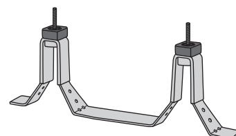
二重葺 断熱金具150
