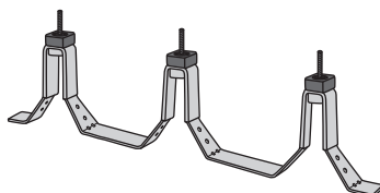
二重葺 断熱金具88
