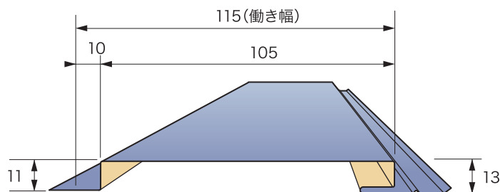
製品図 KBスパン108
