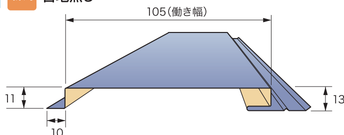
製品図 KBスパン105
